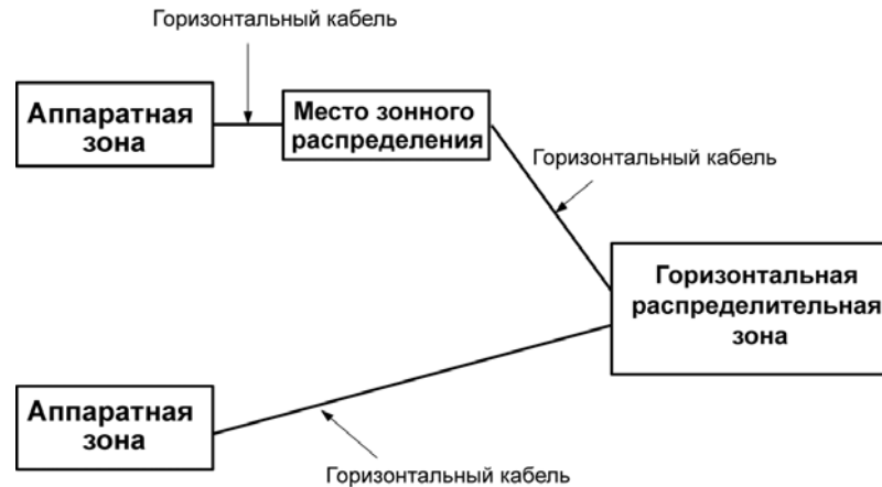
Рис. 7. Типовая схема горизонтальной кабельной разводки с топологией звезды
