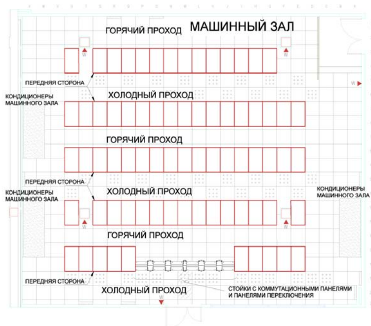
Рис. 20. Схема планировки машинного зала с указанием «горячих» и «холодных» проходов
