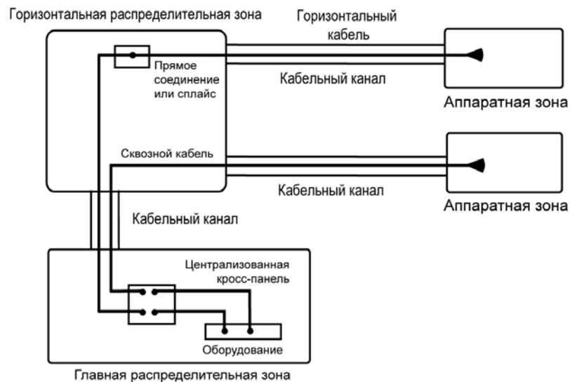
Рис. 9. Централизованная оптическая кабельная разводка
