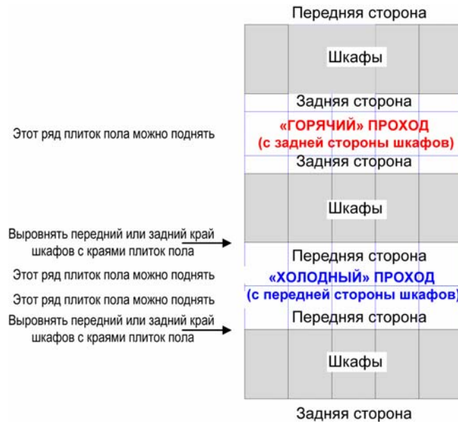
Рис. 6. Пример «горячих» проходов, «холодных» проходов и размещения шкафов
